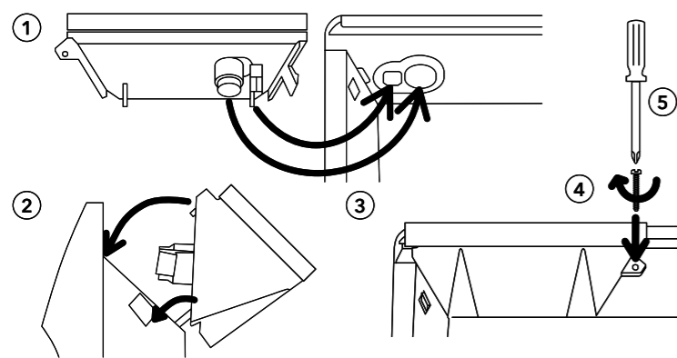
Рис. 3 Схема установки
